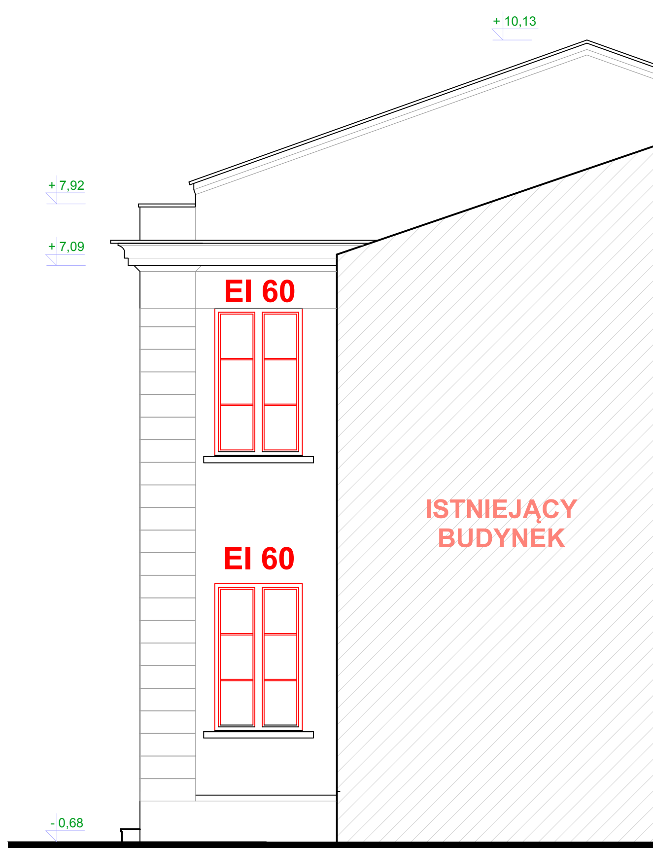
ELEWACJA POŁUDNIOWO-WSCHODNIA
